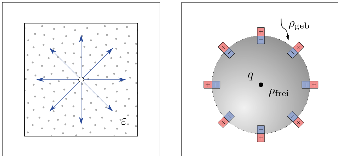
(a) Eine in einem Dielektrikum eingeschlossene Punktladung.
