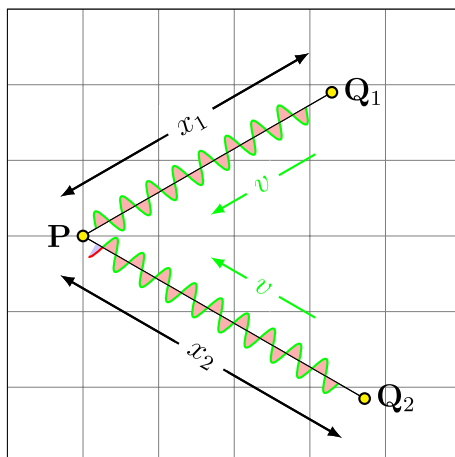
Abbildung 1.19: Gangunterschied.
