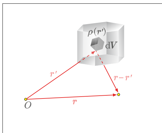
Abbildung 2.5: Ausgedehnte Ladungsverteilung.
