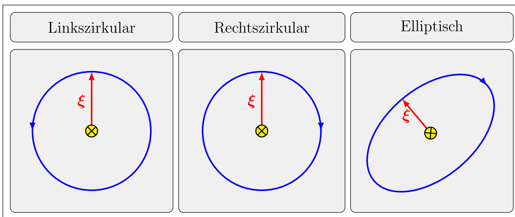
Abbildung 1.12: Zirkulare und elliptische Polarisation.
