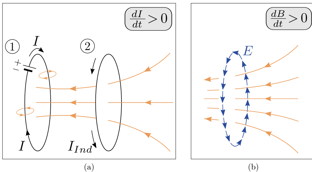
Abbildung 8.8: Eine Erhöhung des Stromes \frac{dI}{dt} > 0 in Leiterschleife 1 induziert ein ringförmiges elektrisches Feld in Leiterschleife 2, welches einen Strom I_{ind} erzeugt, der nun der Flussänderung ( \frac{\partial B}{\partial t} > 0 ) entgegenwirkt.
