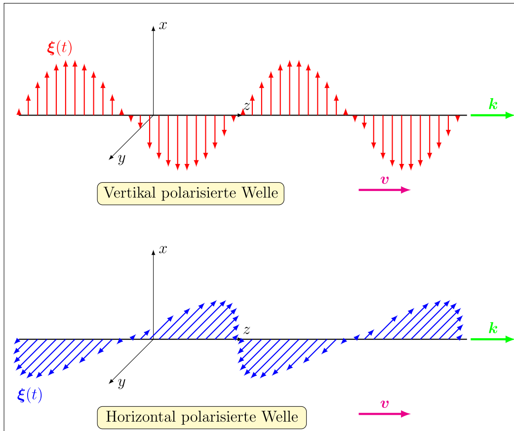
Abbildung 1.11: Horizontal bzw. vertikal polarisierte Welle.
