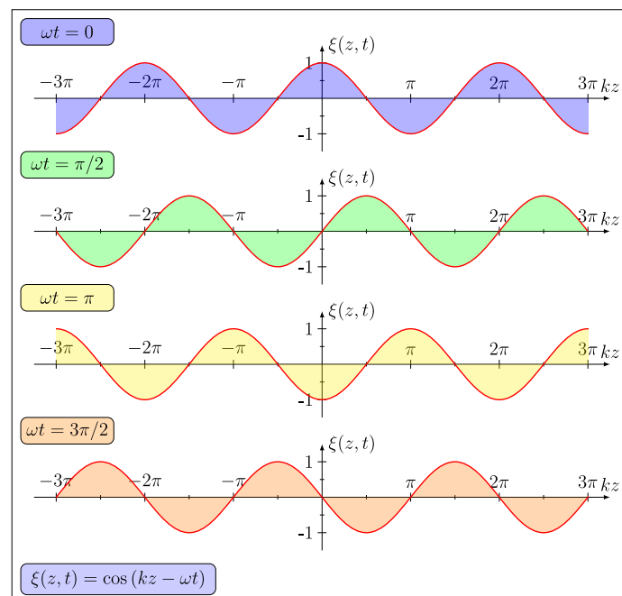
Abbildung 1.15: Ortsabhängigkeit der transversalen Welle für 4 verschiedene Zeitpunkte im abgestuften Abstand von jeweils \Delta t = T/4 .
