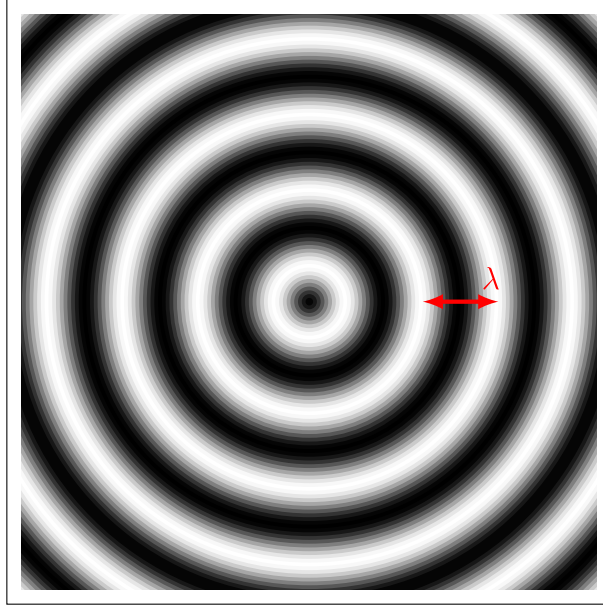
Abbildung 1.13: Longitudinale Kugelwellen.
