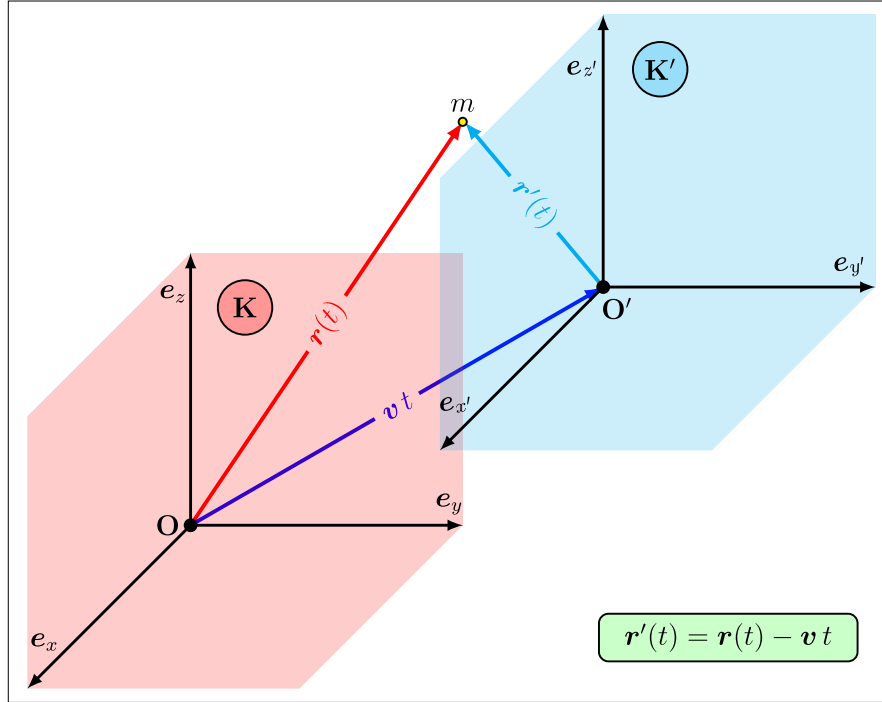
Abbildung 5.2: Der Ort des Massenpunkts m werde in 2 Inertialsystemen beschrieben: Das System K' bewege sich mit der konstanten Geschwindigkeit \mathbf{v} relativ zu K .
