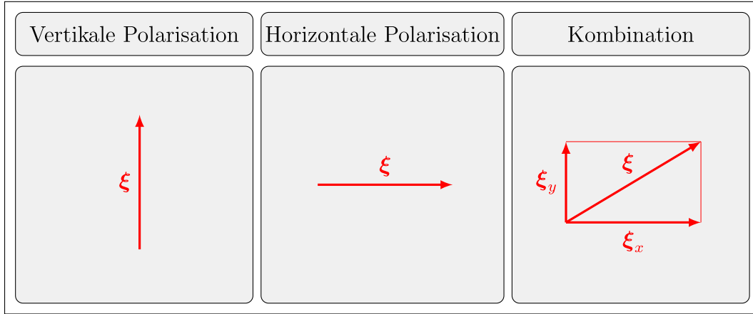
Abbildung 1.10: Lineare Polarisation.
