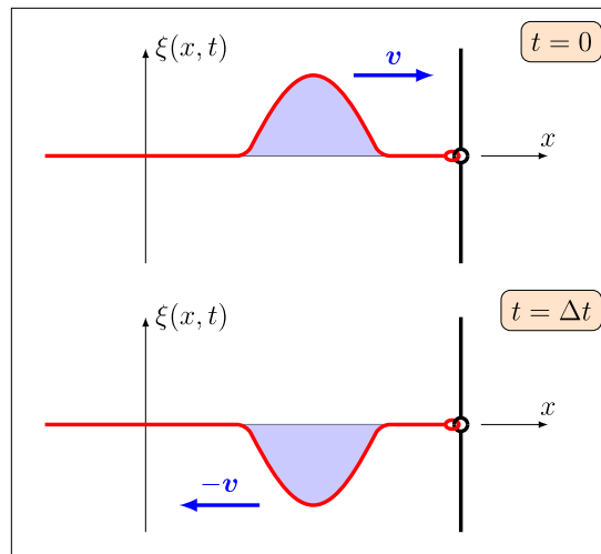
Abbildung 1.22: Reflexion eines Wellenberges am festen Ende.
